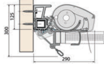
Polaris Sunflex-kulmansäädöllä
